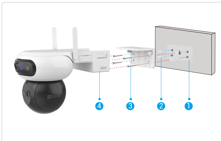
Obr. 2 Montáž na zed'
